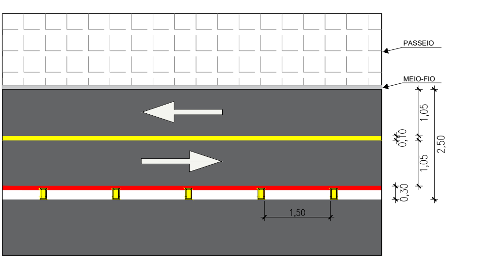
5 TACHÃO REFLETIVO MONODIRECIONAL SEM ESCALA
