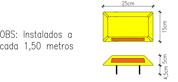
2 TACHÃO REFLETIVO MONODIRECIONAL SEM ESCALA
