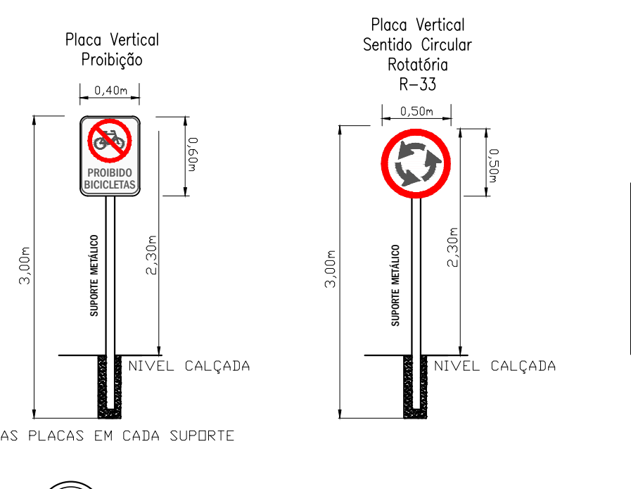
8 SINALIZAÇÃO VERTICAL SEM ESCALA
