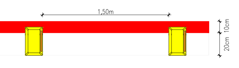
3 DETALHE BORDOS DE PISTA DE CAMINHADA SEM ESCALA
