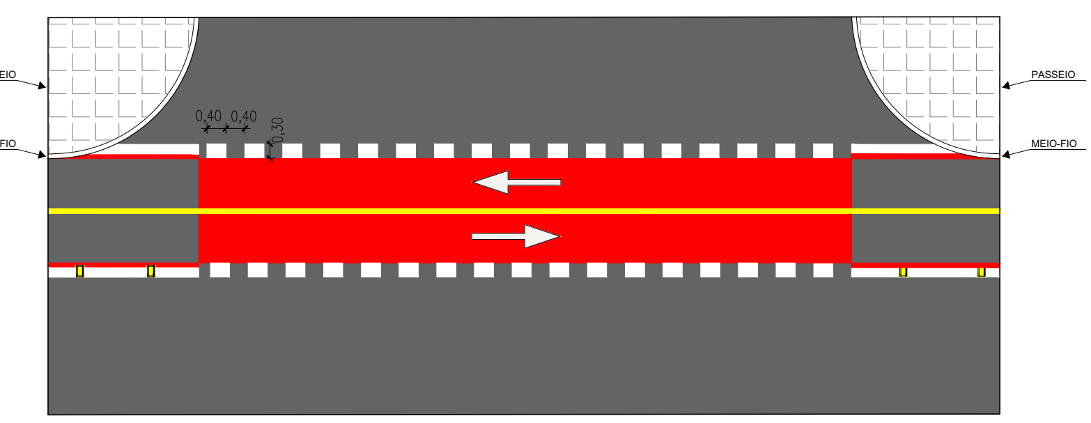
6 DETALHE CRUZAMENTO SEM ESCALA
