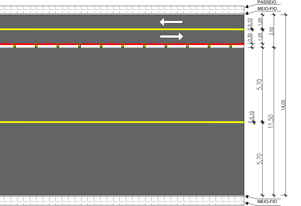
7 DETALHAMENTO GERAL SEM ESCALA
